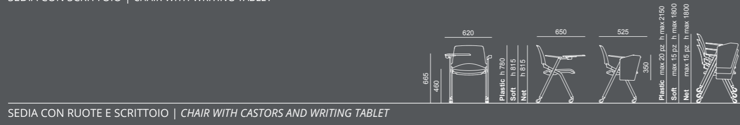
SEDIA CON SCRITTOIO | CHAIR WITH WRITING TABLET
