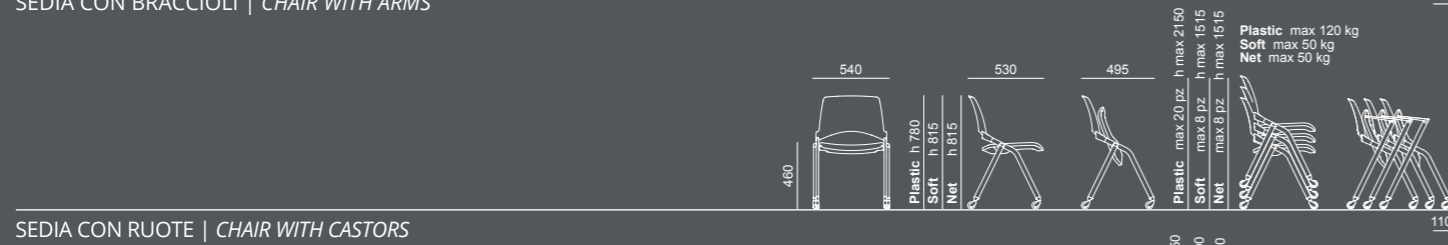
SEDIA CON BRACCIOLI | CHAIR WITH ARMS
