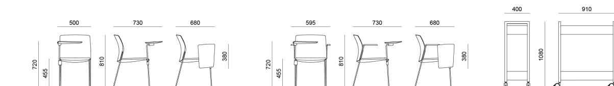
Sedia trapezio con scrittoio + carrello porta tavolette / Skid chair with writing tablet + trolley for writing tablets
