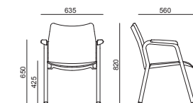
SEDIA CON POGGIA BRACCIA - CHAIR WITH ARMREST PADS
