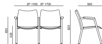
PANCA CON POGGIA BRACCIA - BENCH WITH ARMREST PADS
