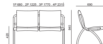
PANCA CON SCHIENALE - BENCH WITH BACKREST
