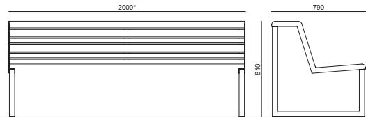
PANCA CON SCHIENALE E DOPPIA SEDUTA - DOUBLE SEAT WITH BACKREST
