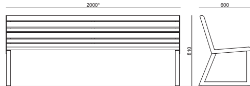
PANCA CON SCHIENALE - SEAT WITH BACKREST
